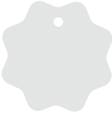
PEN038-R2 f.to: mm 58x58 f.to foro: Ø mm 5
