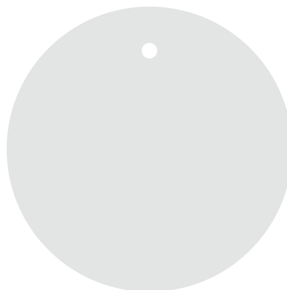
PEN016-R4 f.to: Ø mm 55 f.to foro: Ø mm 3
