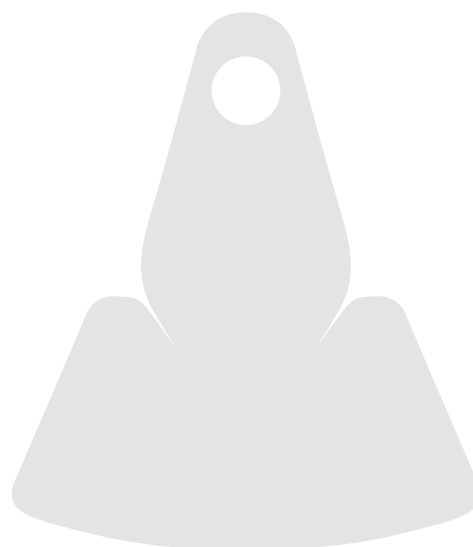
PEN022-R2 f.to: mm 62x70 f.to foro: Ø mm 10
