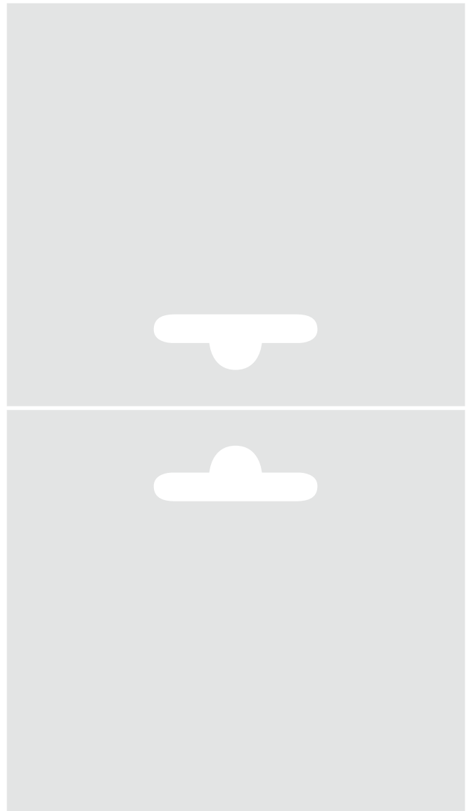
PEN035-R1 Fori e cordonatura per pendagli f.to base: mm 85 f.to altezza: misura variabile f.to foro: mm 30x10
