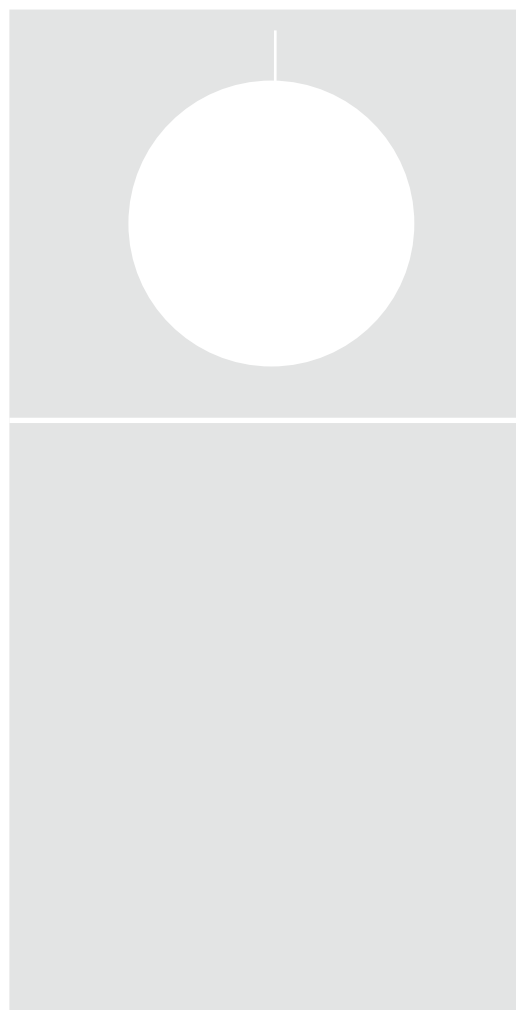
PEN028-R1 Pendaglio cordonato f.to: mm 68x133 f.to foro: Ø ≥ mm 38
