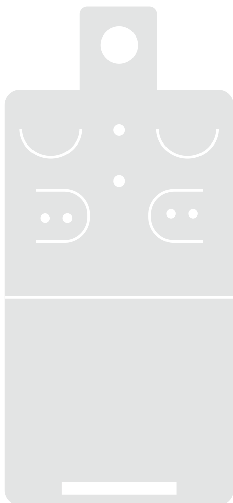
PEN024-R2 Pendaglio cordonato f.to aperto: mm 60x130 f.to chiuso: mm 60x54 + linguetta aggancio mm 20x21 f.to foro: Ø mm 10
